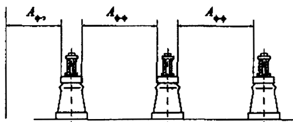
Рис. 4.2.14. Наименьшие расстояния в свету между неизолированными токоведущими частями разных фаз в ЗРУ и между ними и заземленными частями (по табл. 4.2.9 )
